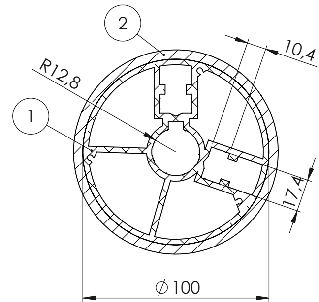
SEZIONE A-A
